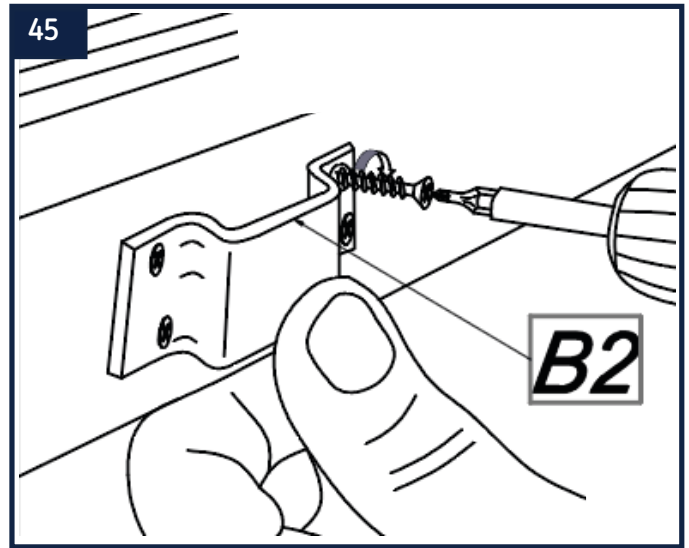
Fixez ensuite une première gâche (B2) sur la margelle extérieure courte (12) à l'aide des vis 4 x 40 mm (F).
