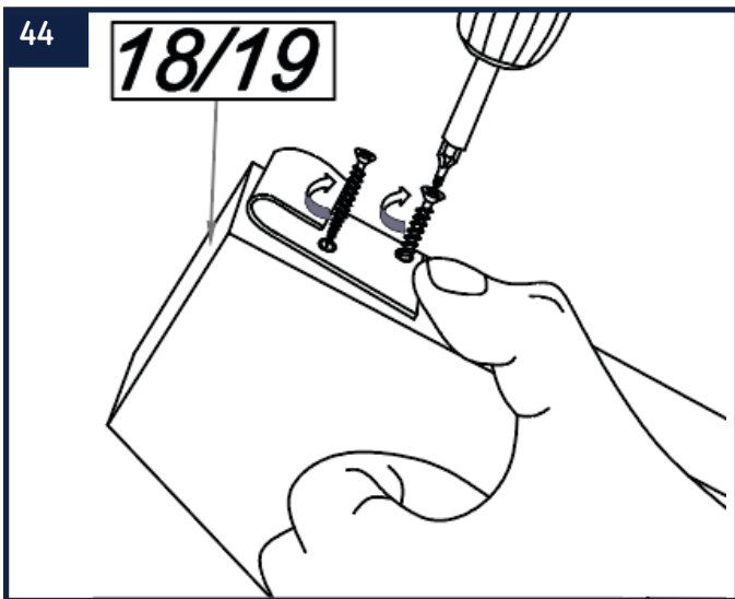
Fixez les boucles de l'échelle (B1) sur les limons gauche (18) et droite (19) de l'échelle à l'aide des vis 4 x 40 mm (F).
